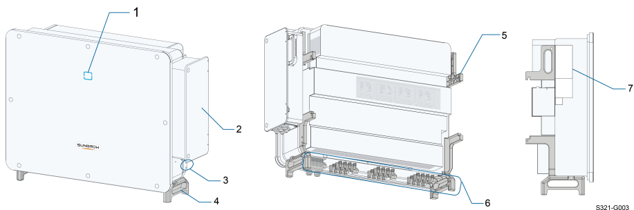
figure 2-2 Apparence de l'onduleur
