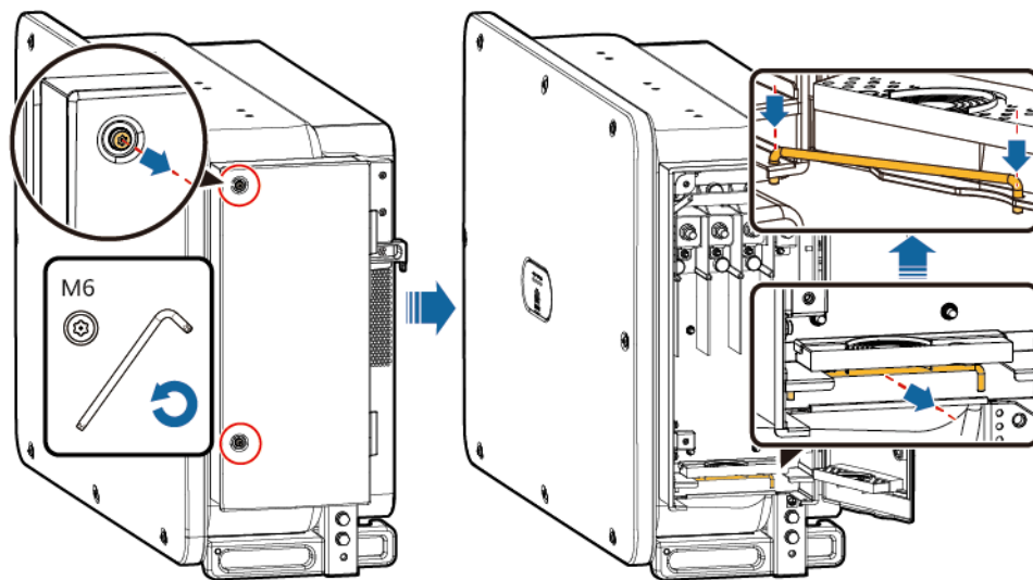
Figure 5-5 Ouverture de la porte du compartiment de maintenance
