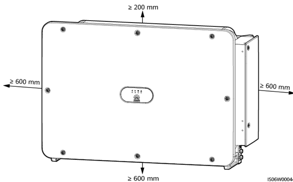
Figure 4-2 Espace d'installation
