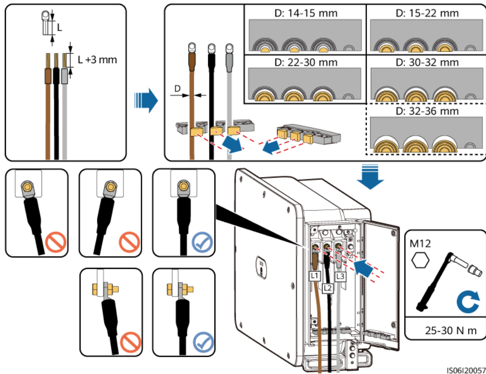
Figure 5-13 Connexion de câble
