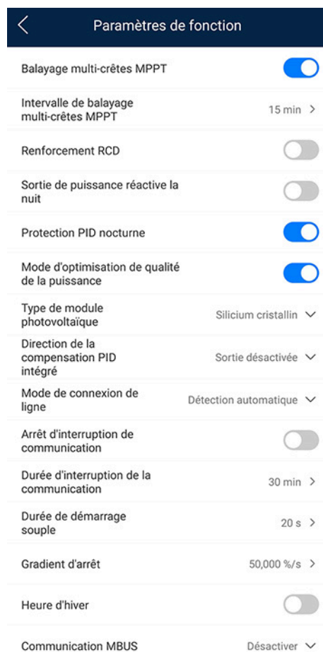
Figure 7-3 Paramètres de fonction (Utilisateur avancé)
