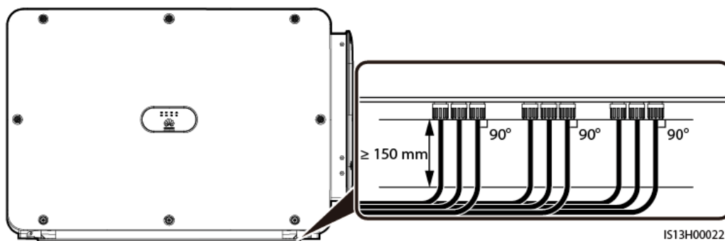
Figure 5-19 Exigences en matière de câblage d'alimentation d'entrée CC
