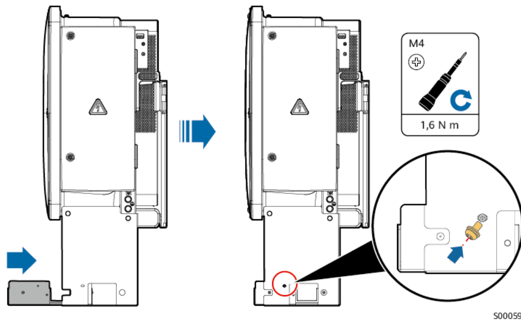
Figure 4-16 Installation du panneau inférieur
