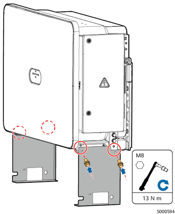
Figure 4-15 Installation des panneaux latéraux
