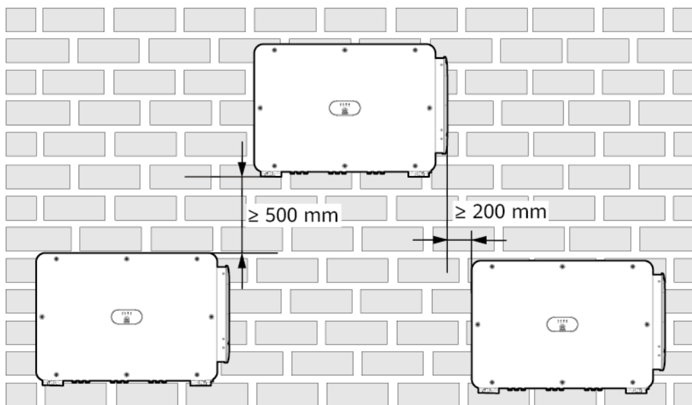
Figure 4-5 Mode d'installation en triangle (recommandé)
