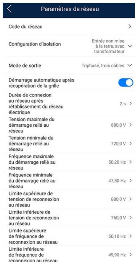
Figure 7-4 Paramètres de réseau (Utilisateur spécial)
