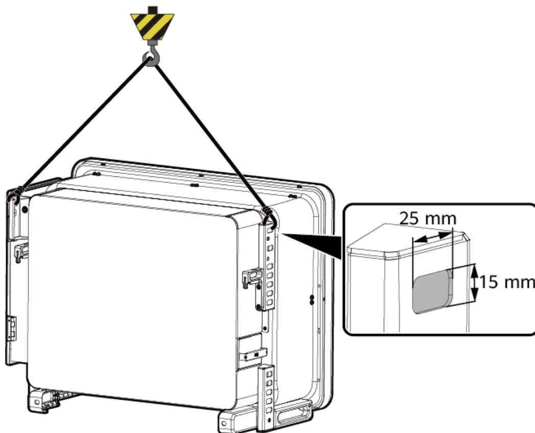
Figure 4-14 Levage de l'onduleur
