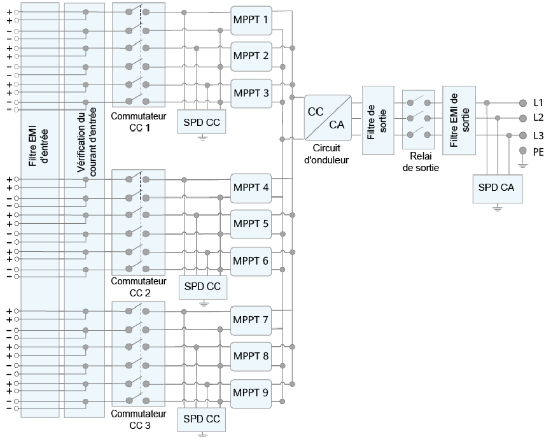
Figure 2-7 Schéma conceptuel de l'onduleur
