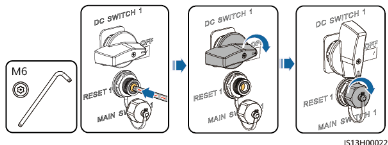
Figure 8-17 Réinitialisation et mise sous tension du commutateur C (DC SWITCH 1 est utilisé comme exemple)
