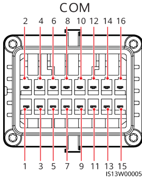
Figure 5-18 Définitions des broches
