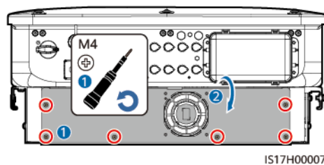
Figure 8-2 Dépose de la plaque de déflecteur de la grille d'entrée d'air
