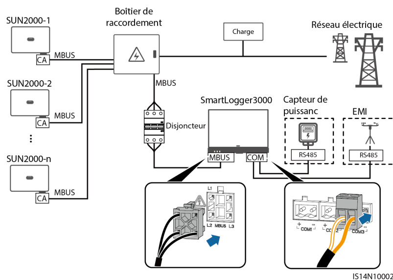
Figure 5-23 Communication MBUS (scénario C&I en Chine)
