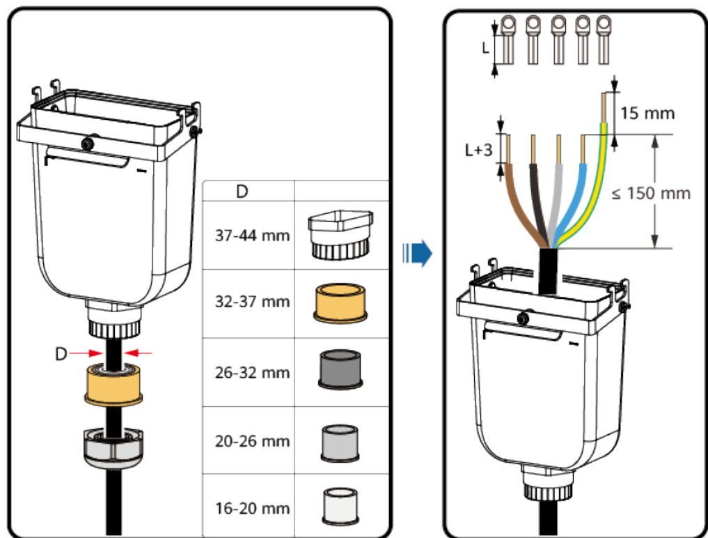
Figure 5-6 Dénudez le câble d'alimentation CA (un câble à cinq conducteurs sert d'exemple).
