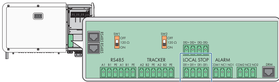
Figure 9 : Entrées numériques pour la fonction d'arrêt rapide sur l'ensemble COM
